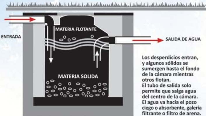
NUESTRA CÁMARA SÉPTICA
